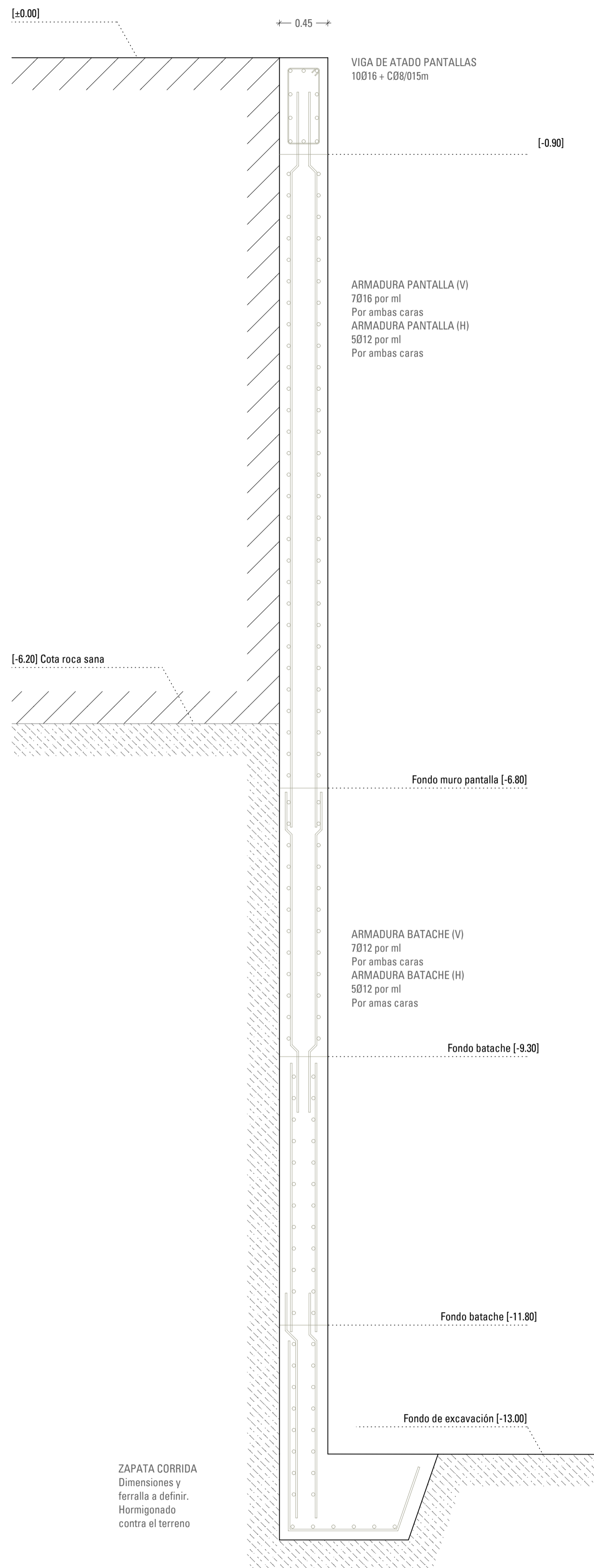
DETALLE TIPO 1 Contención contra el terreno
