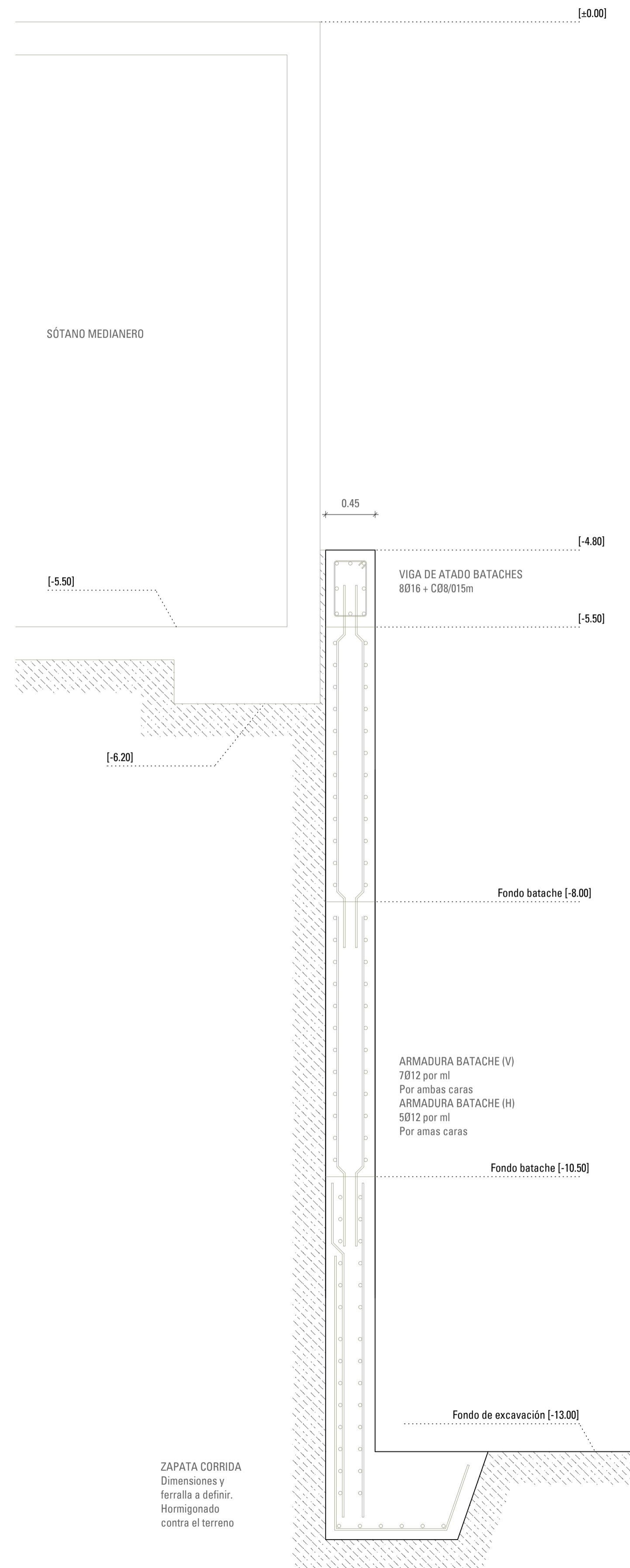
DETALLE TIPO 2 Contención contra sótano medianero
